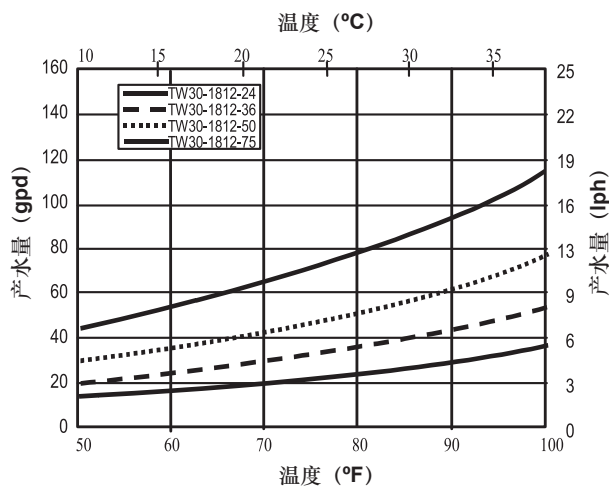
图 2 温度对产水流量的影响 (固定压力和回收率)
