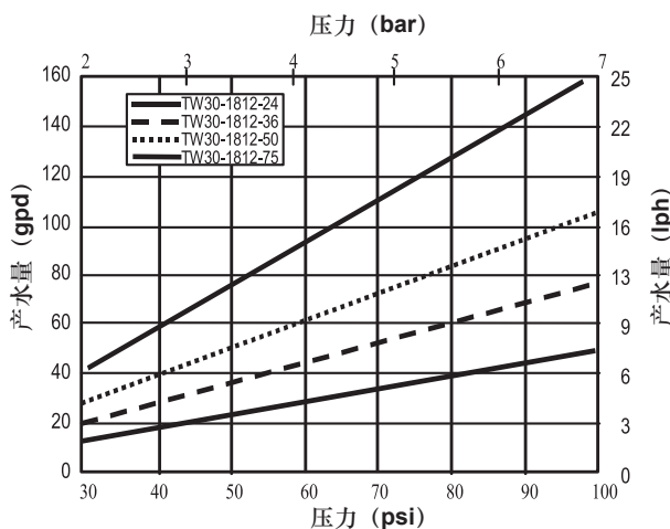
图 1 压力对产水流量的影响 (固定温度和回收率)
